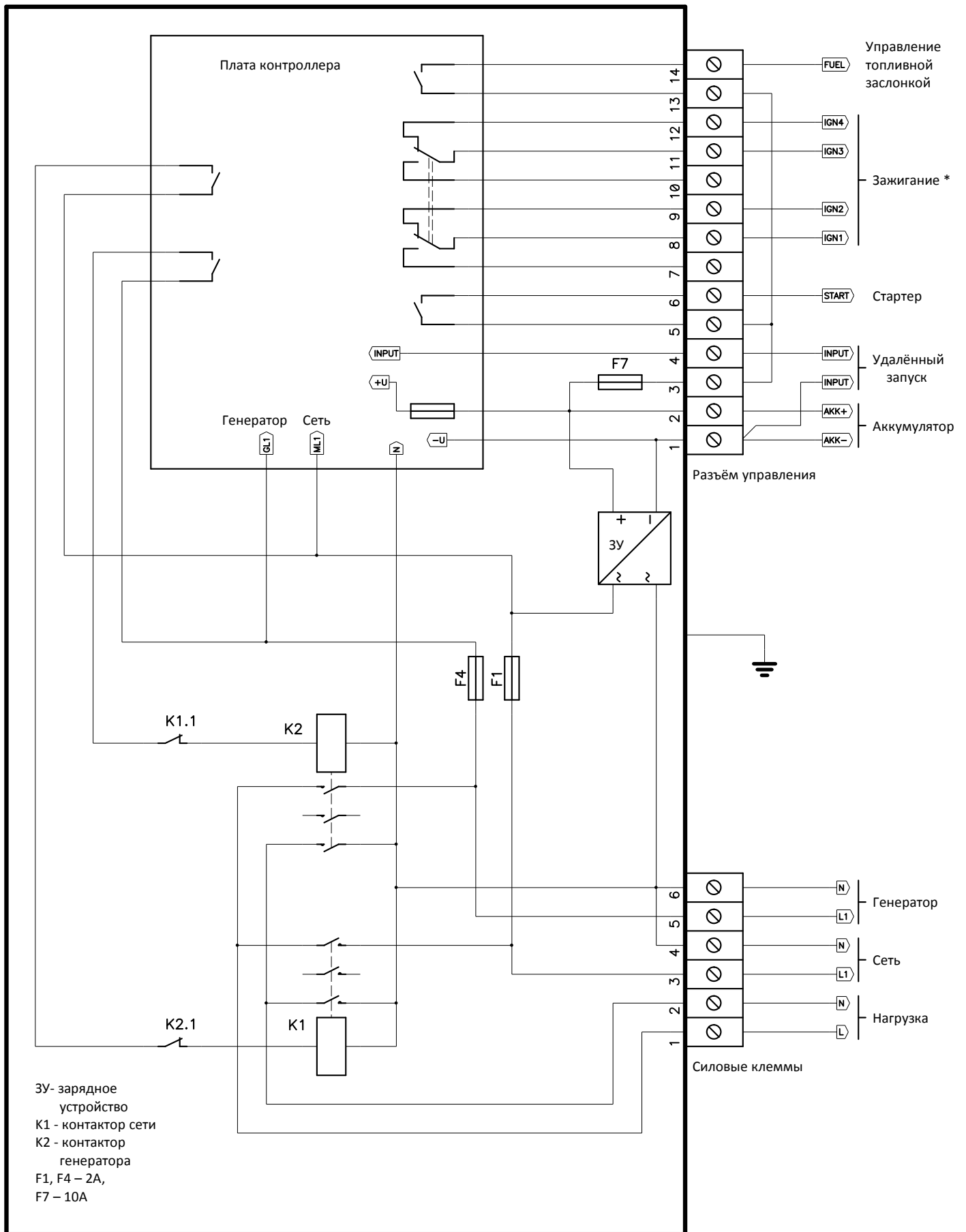
Рис 6.2. Пример схемы подключения контроллера АВР11МЕ / АВР11СЕ.
