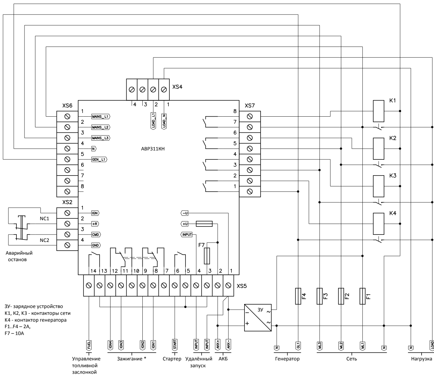
Рис 6.2. Пример схемы подключения контроллера AVR311KH.
