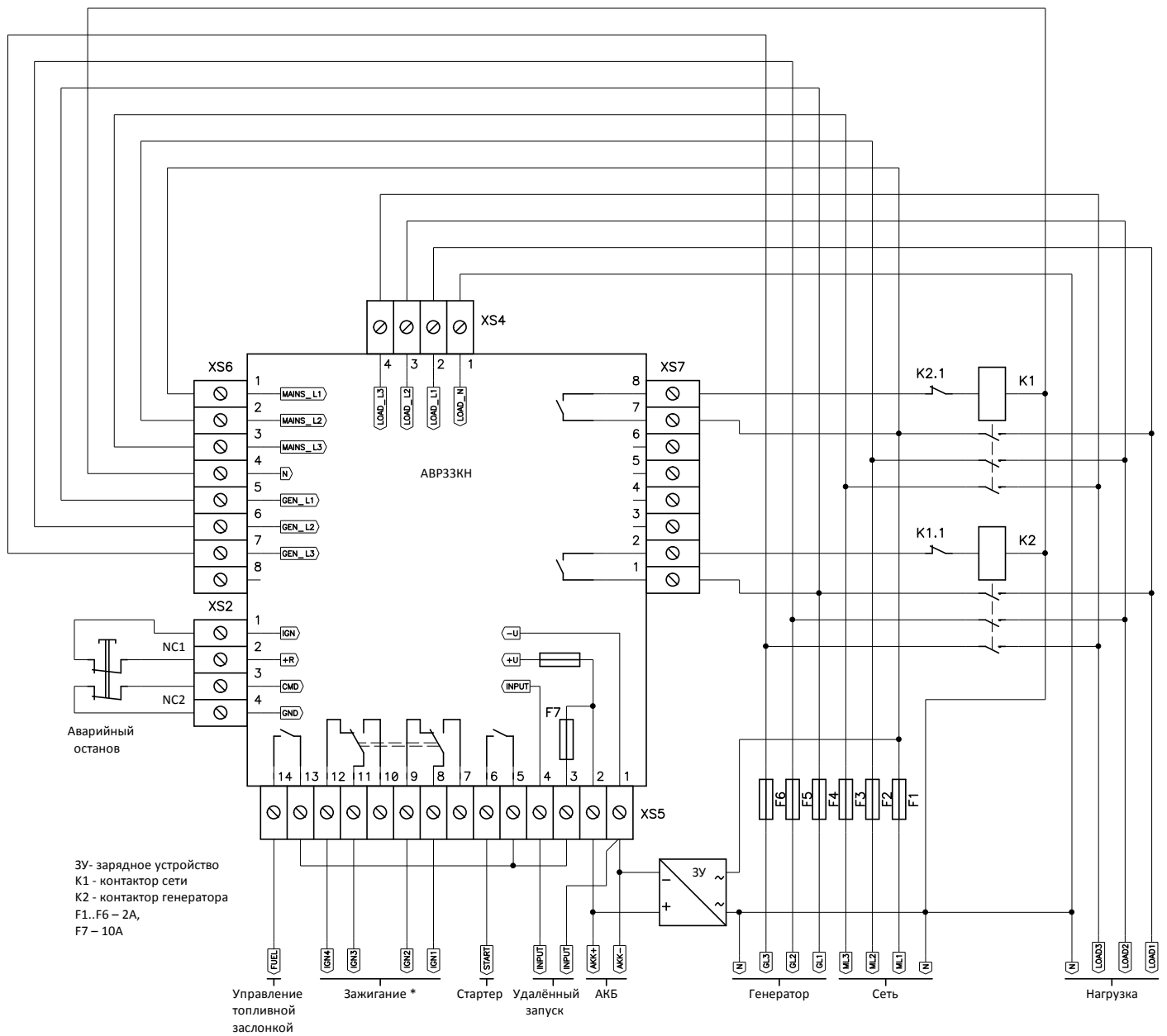
Рис 6.2. Пример схемы подключения контроллера AVR33KH.
