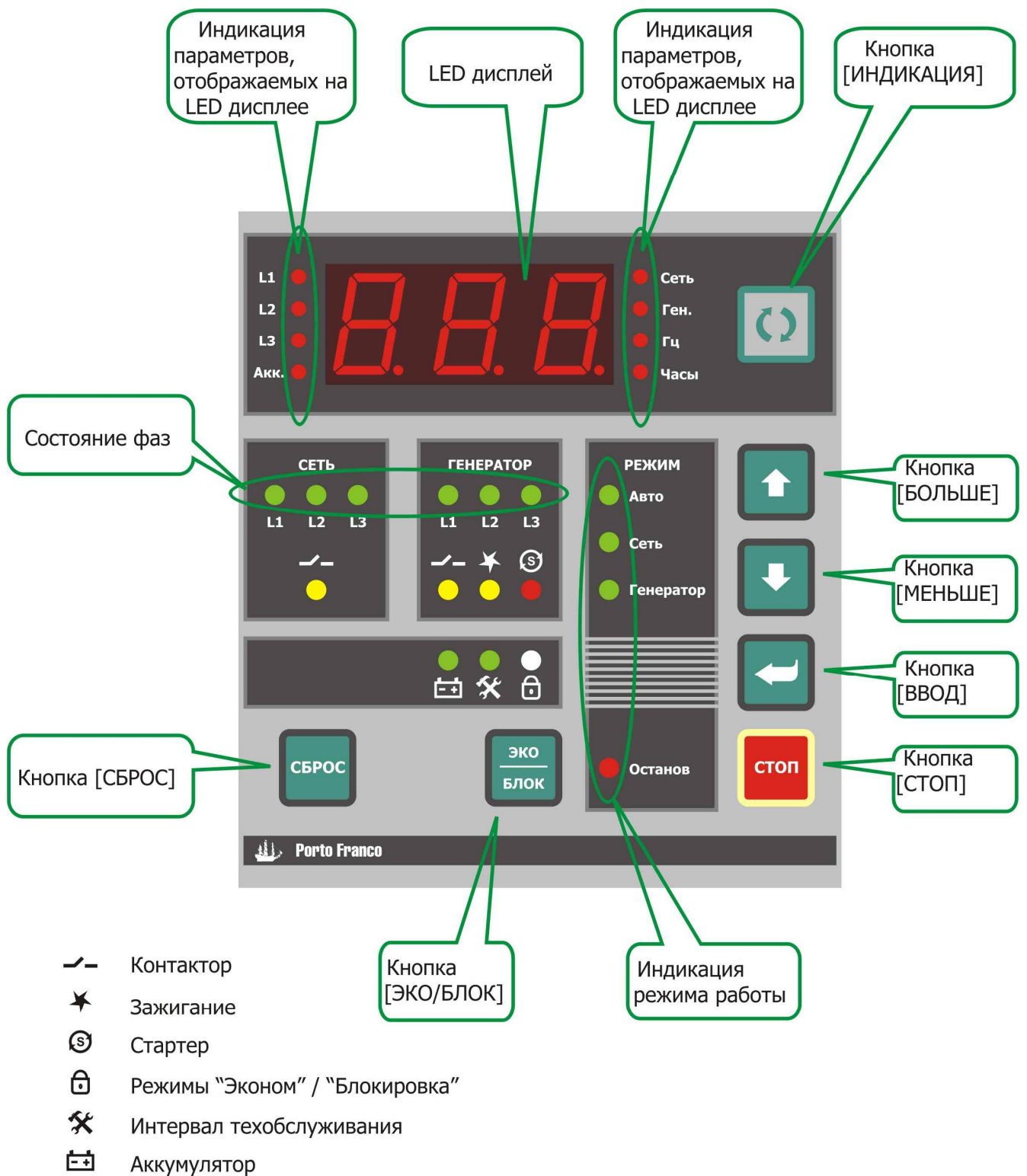
Рис. 5.2. Панель индикации и управления
