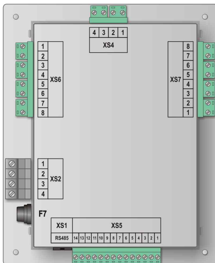
Рис 6.1. Клеммы и разъёмы подключения контроллера (вид сзади).
