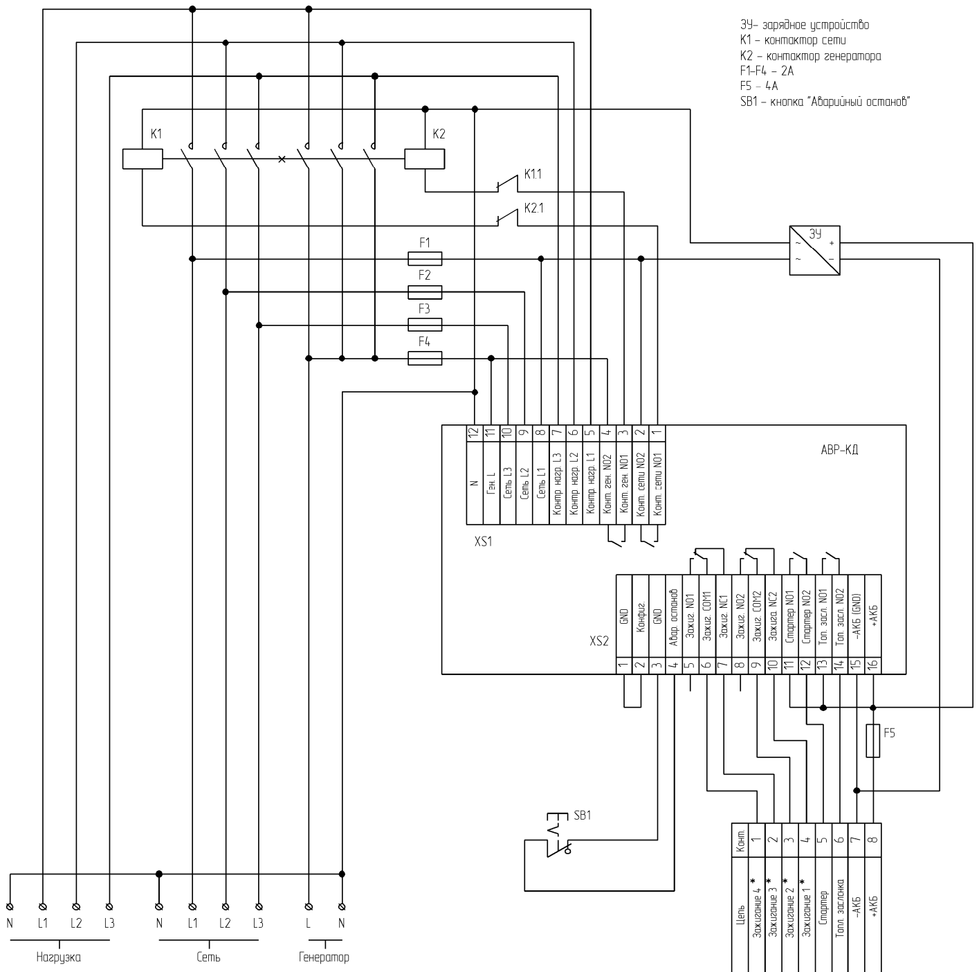
Рис 6.2. Пример схемы подключения контроллера AVR-КД для трёхфазной сети
