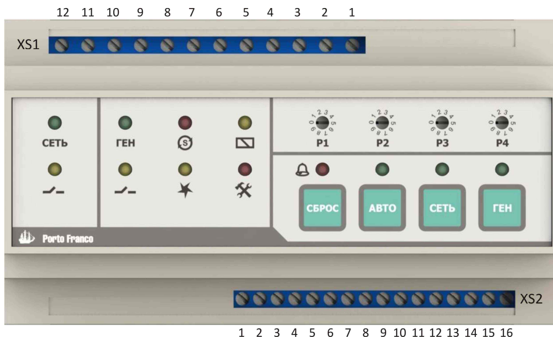
Рис 6.1. Клеммы подключения АВР-КД
