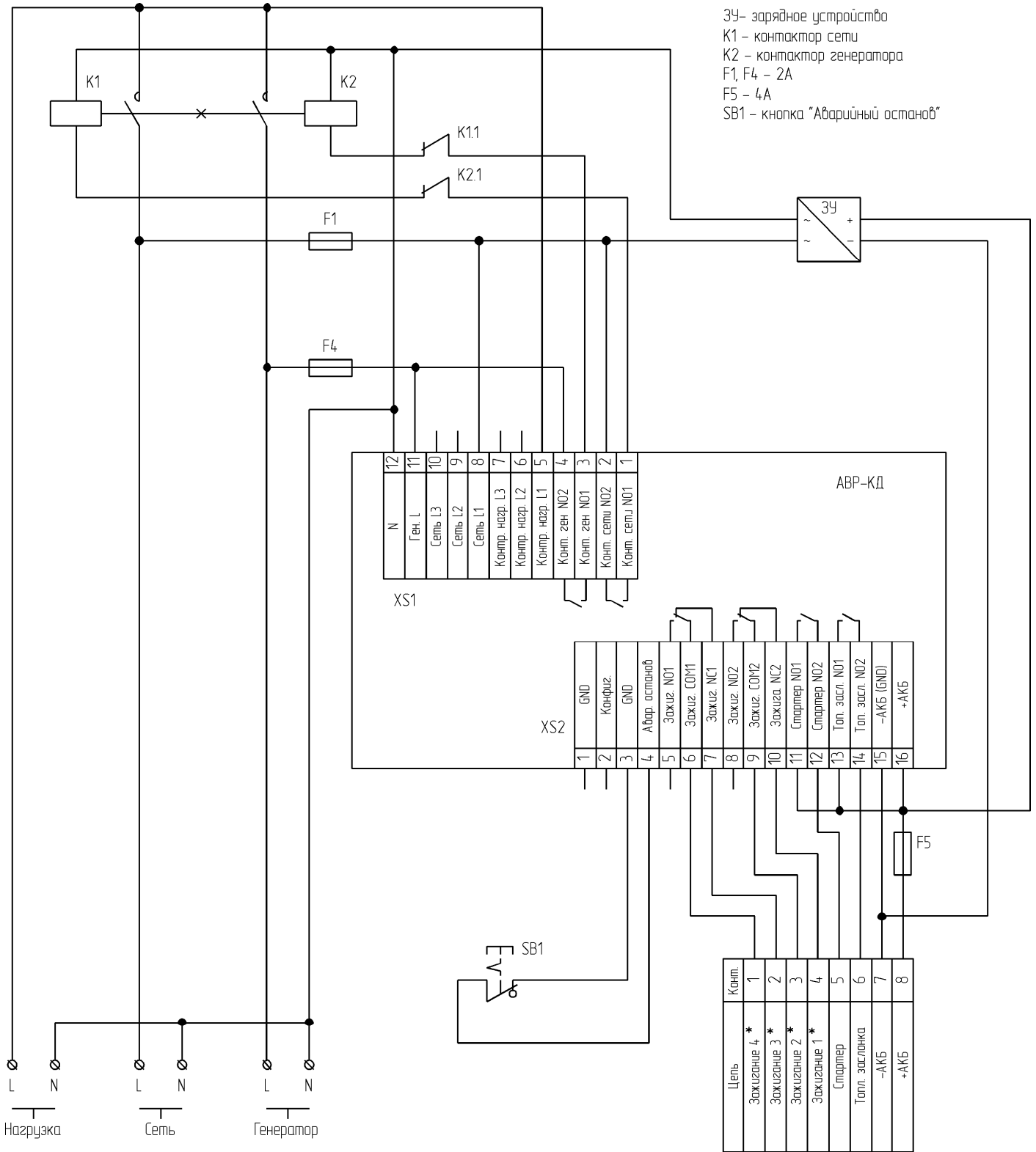
Рис 6.3. Пример схемы подключения контроллера AVR-КД для однофазной сети
