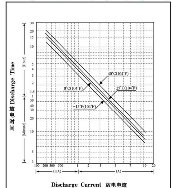
放电特性 Discharge Characteristics(0°C/32°F,40°C/104°F)
