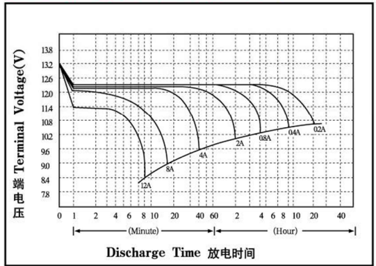
放电特性 Discharge Characteristics(20°C,68°F)
