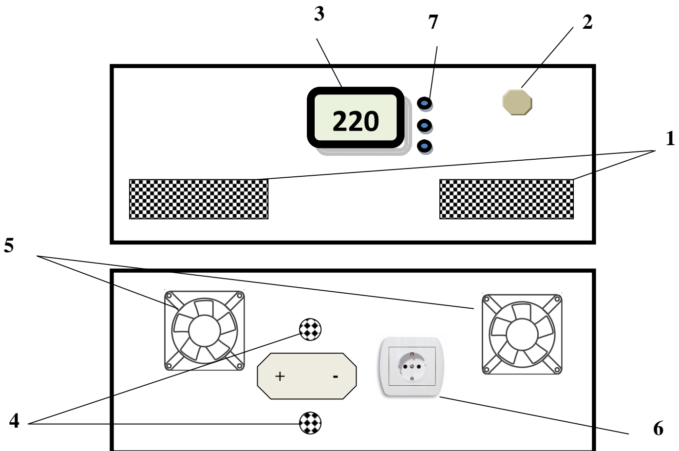
Рис.1. Передняя и задняя панель ИБП, где: 1 – вентиляционные отверстия, 2- кнопка управления ИБП, 3 – жидкокристаллический дисплей, 4 – разъем для подключения АКБ, 5 – система охлаждения, 6 –розетка с заземлением для подключения нагрузки не более 500Вт, 7 – индикаторы готовности.
