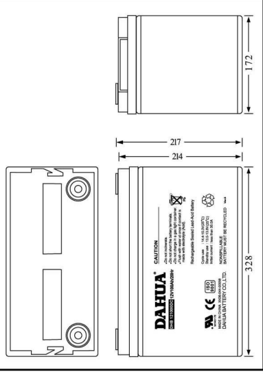
Dimensions 尺寸 (mm)
